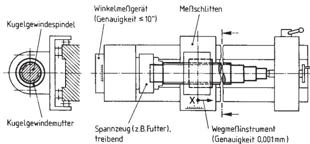
Bild 1. Meßprinzip
